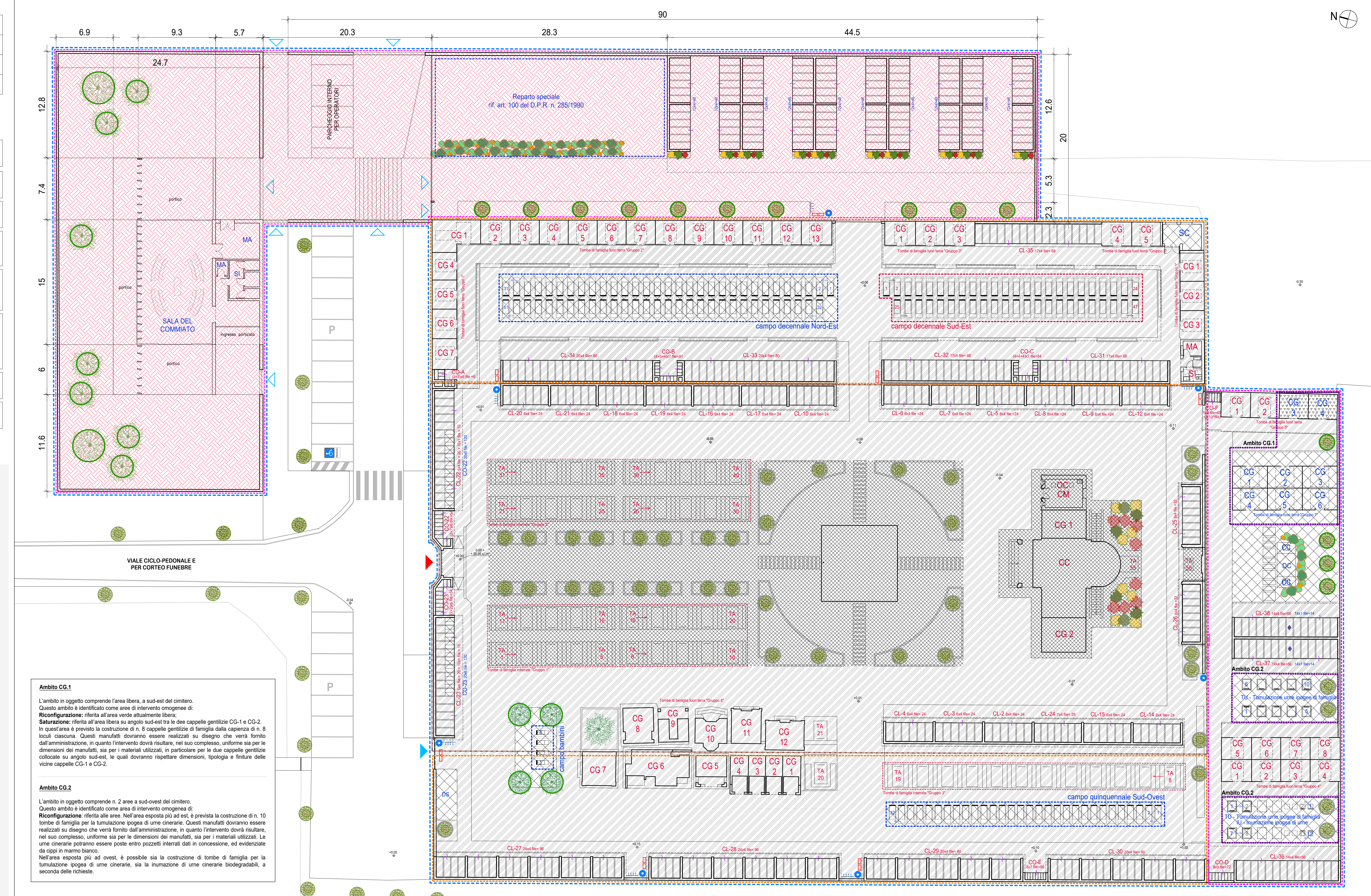
PLANIMETRIA GENERALE - INDIVIDUAZIONE AREE DI INTERVENTO OMOGENEE - Scala 1:200
